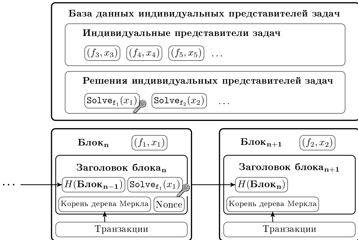
Рис. 2: Модель разработанного UPoWB-блокчейна. Рисунок иллюстрирует невозможность формирования n + 1 блока, так как ассоциированная с ним задача еще не прошла проверку администратором базы данных индивидуальных представителей полезных задач
