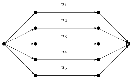
Рис. 4. Сеть G_1
