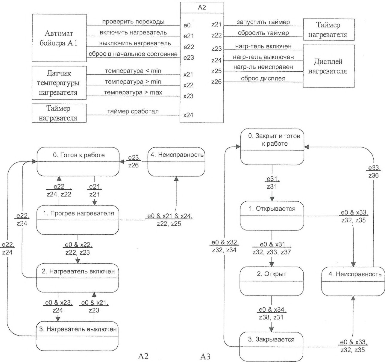
Автомат управления нагревателем
